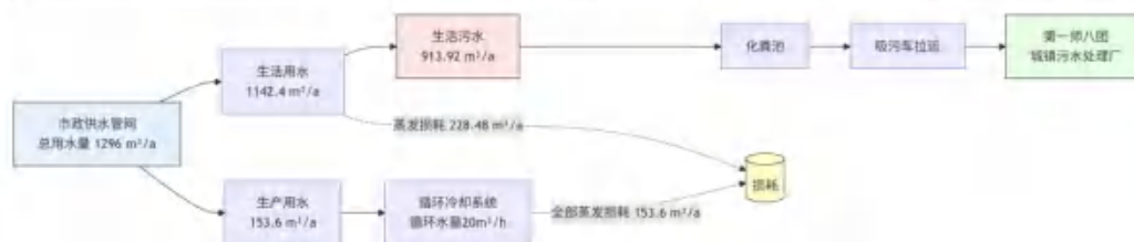
图 2-1 项目营运期水平衡单位: m 3 /a
