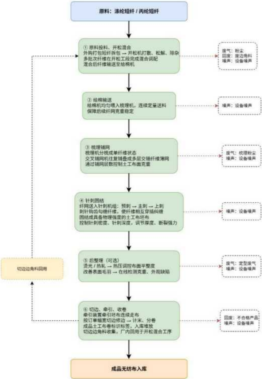
图 2-3 无纺布工艺及产污环节
