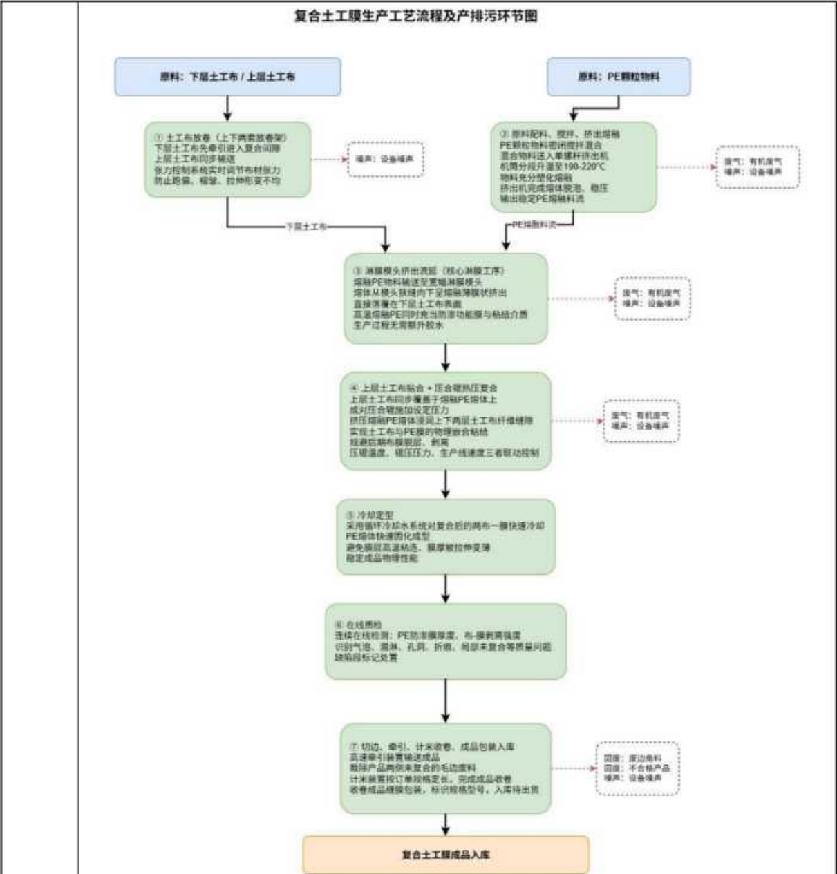
图 2-4 复合土工膜工艺及产污环节
