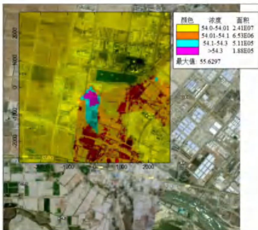
图 5.1.2-2 NO 2 保证率日均叠加浓度分布图
