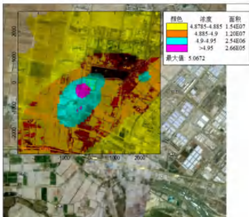
图 5.1.2-4 SO 2 年均叠加浓度分布图
