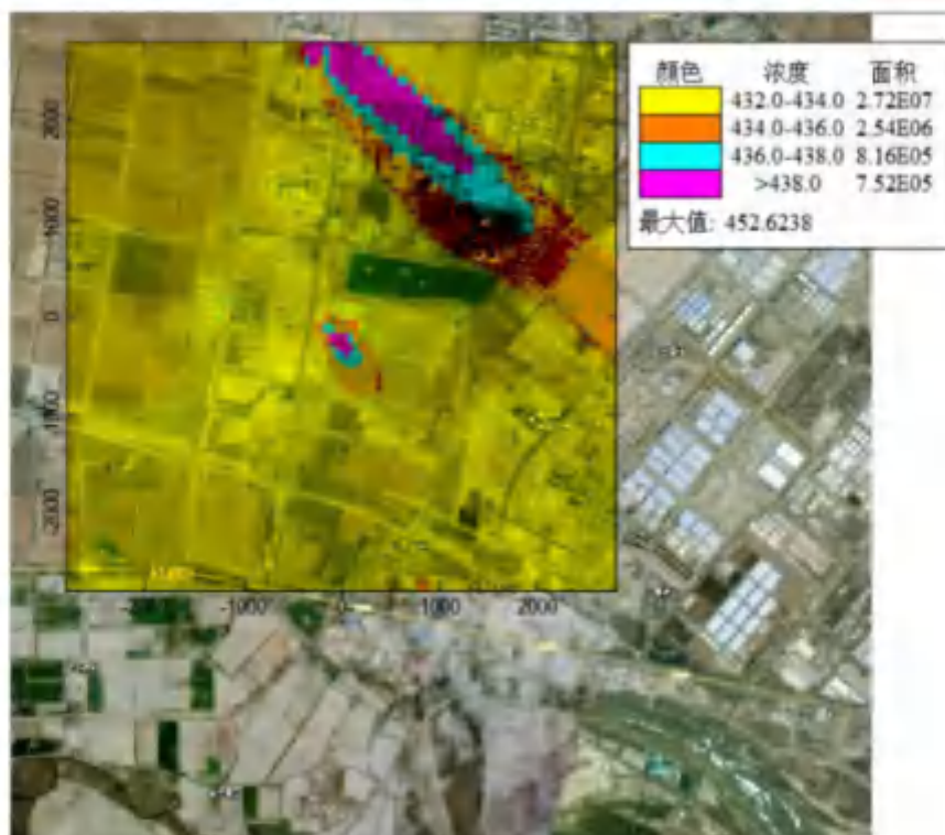
图 5.1.2-3 PM 10 保证率日均叠加浓度分布图
