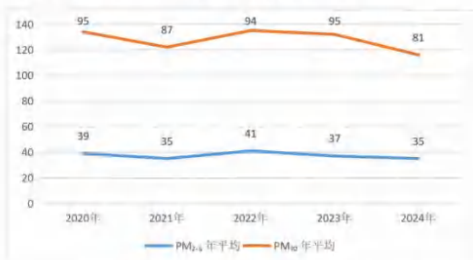
图 4.3.3-1 PM 10 、PM 2.5 年均浓度趋势图 (2020~2024 年)
