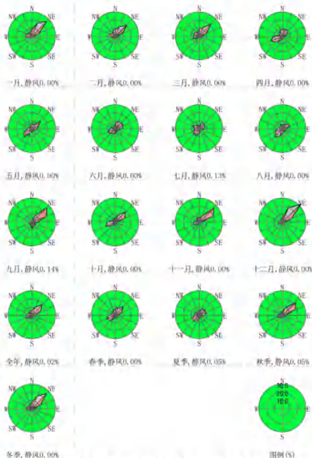
图 5.1.1-1 阿拉尔市气象站 2024 年污染系数玫瑰图
