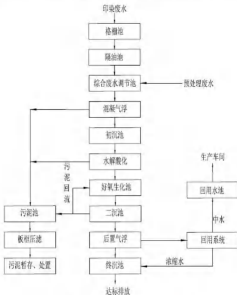
图 6.2.2-3 印染废水处理系统工艺流程
