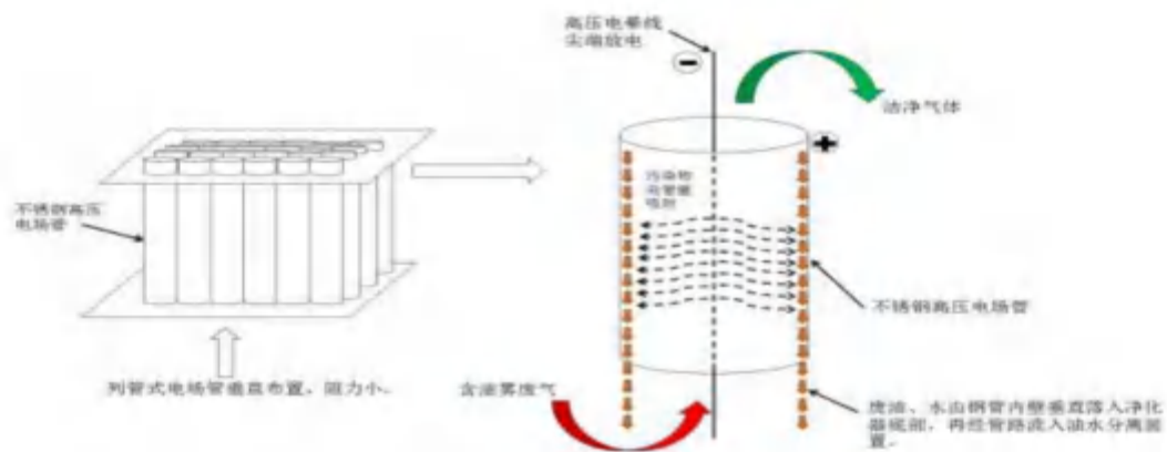
6.1.1-2 静电吸附装置
