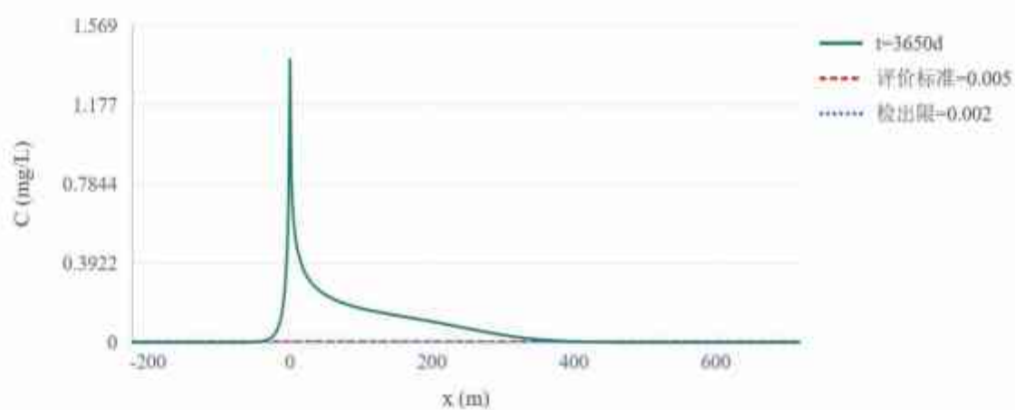
图 5.3.2-36 铅 t=3650d 地下水流向浓度变化趋势图
