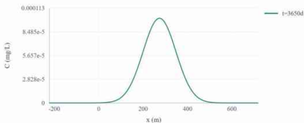
图 5.3.2-18 -镉 t=3650\text{ d} 地下水流向浓度变化趋势图
