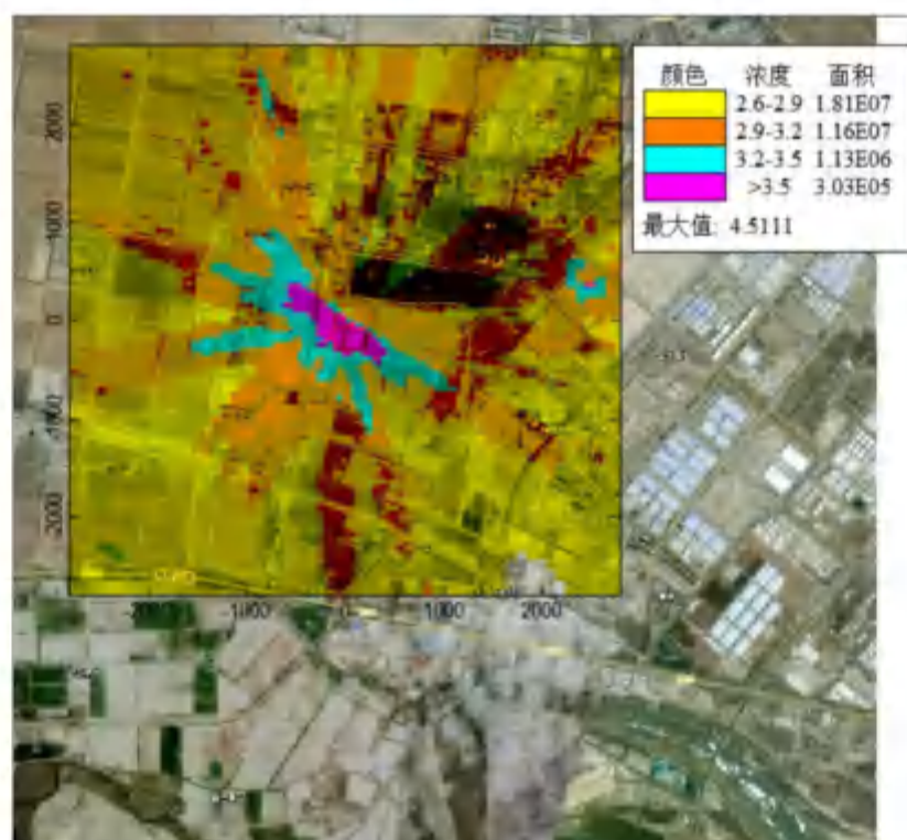
图 5.1.2-8 硫化氢小时叠加浓度分布图
