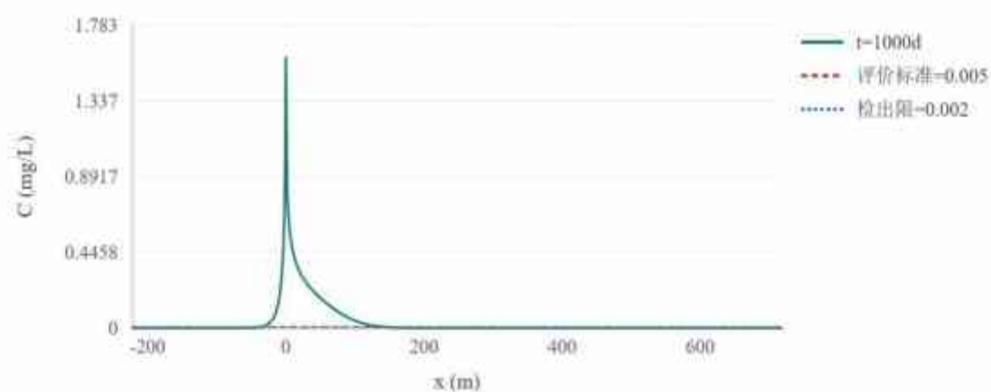
图 5.3.2-34 铅 t=1000d 地下水流向浓度变化趋势图
