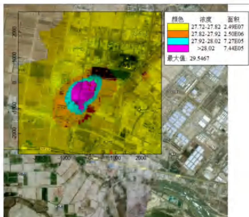
图 5.1.2-5 \text{NO}_2 年均叠加浓度分布图
