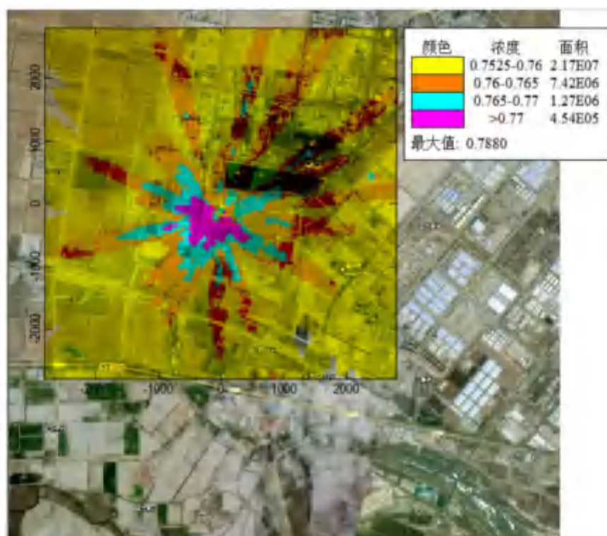
图 5.1.2-12 二甲苯小时叠加浓度分布图
