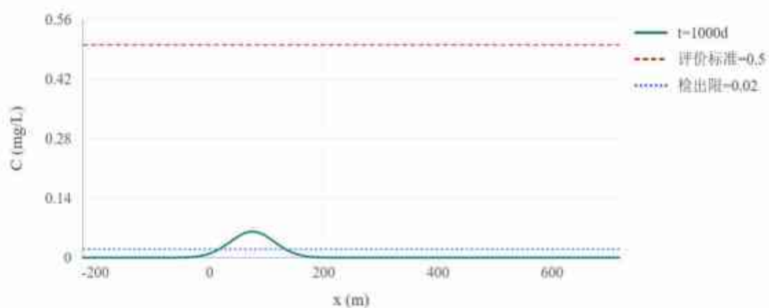
图 5.3.2-10 氨氮（以 N 计） t=1000d 地下水流向浓度变化趋势图
