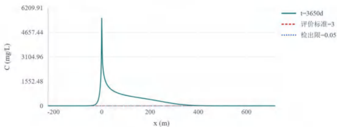
图 5.3.2-24-耗氧量 (COD Mn 法, 以 O 2 计) t=3650d 地下水流向浓度变化趋势图
