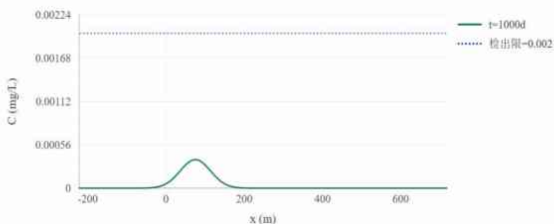
图 5.3.2-16 -镉 t=1000\text{ d} 地下水流向浓度变化趋势图
