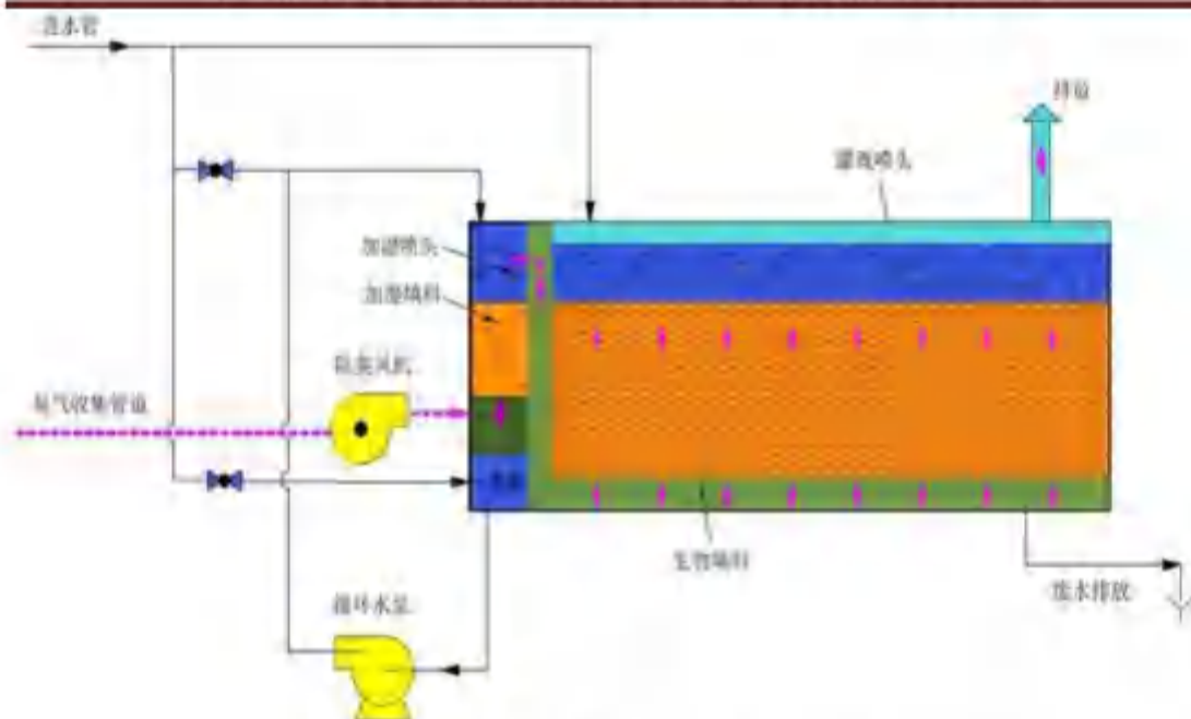
图 6.1.1-4 生物滤池除臭工艺流程
