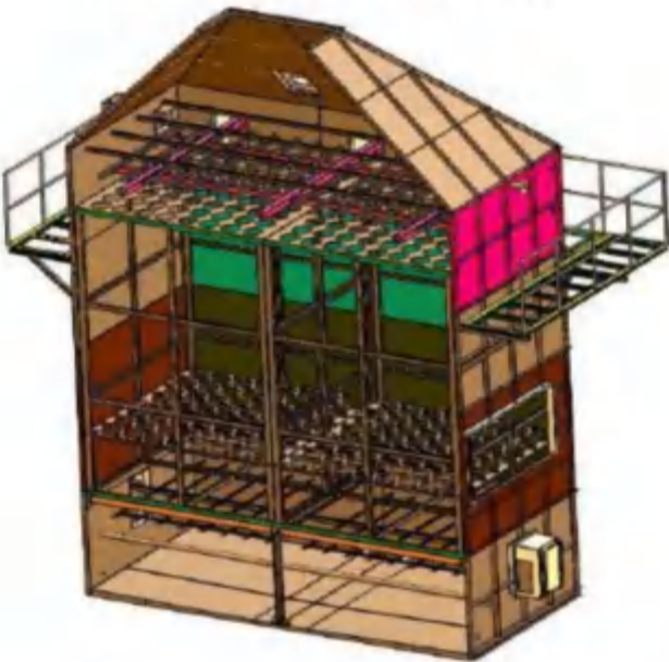
图 6.1.1-3 静电除油内部结构图
