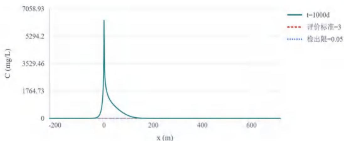
图 5.3.2-22 耗氧量 (COD Mn 法, 以 O 2 计) t=1000d 地下水流向浓度变化趋势图
