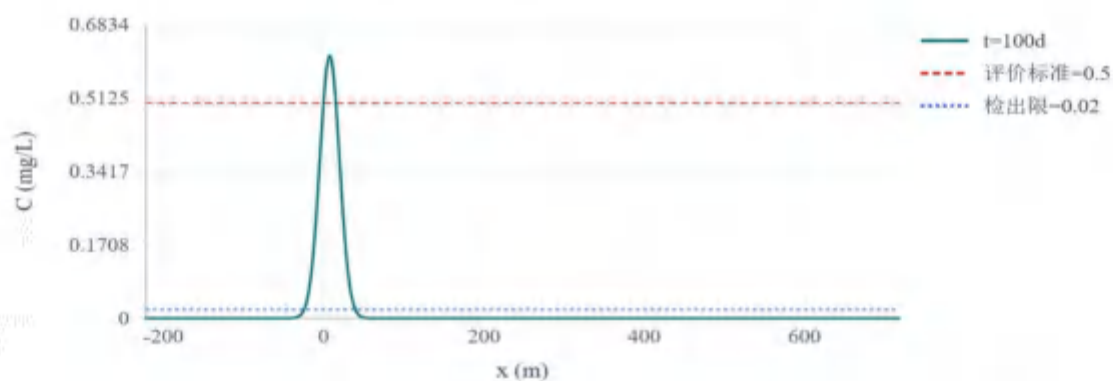
图 5.3.2-8 氨氮（以 N 计） t=100\text{ d} 地下水流向浓度变化趋势图
