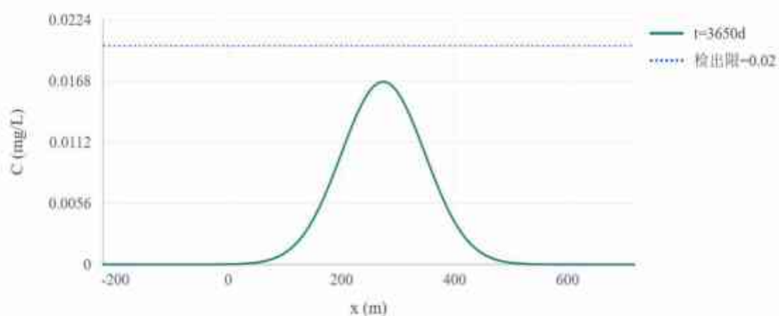
图 5.3.2-12 氨氮（以 N 计） t=3650d 地下水流向浓度变化趋势图
