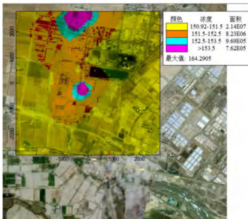
图 5.1.2-6 PM_{10} 年均叠加浓度分布图
