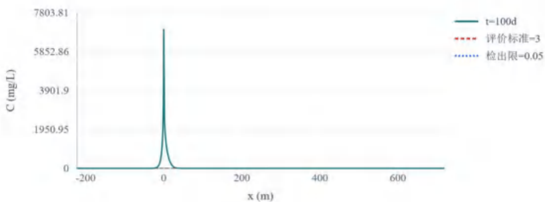
图 5.3.2-20 耗氧量 (COD mn 法, 以 O 2 计) t=100d 地下水流向浓度变化趋势图
