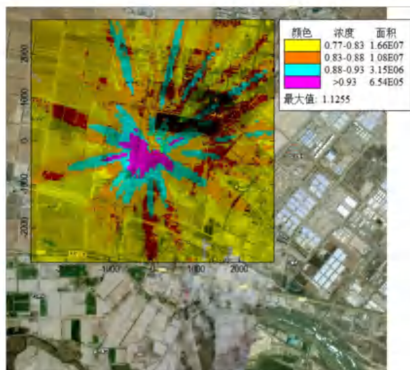
图 5.1.2-11 甲苯小时叠加浓度分布图
