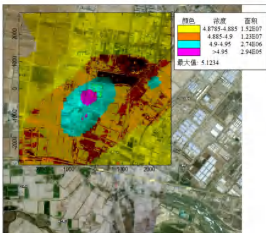
图 5.1.2-4 \text{SO}_2 年均叠加浓度分布图
