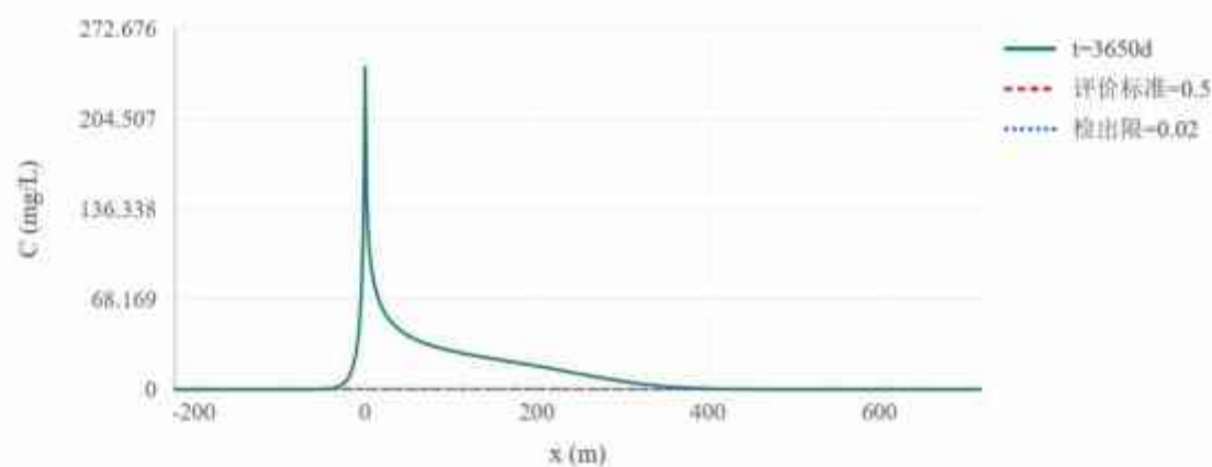
图 5.3.2-30 氨氮（以 N 计） t=3650d 地下水流向浓度变化趋势图
