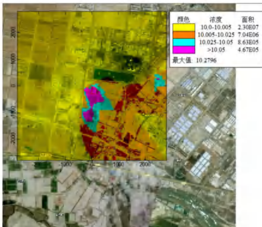
图 5.1.2-1 \text{SO}_2 保证率日均叠加浓度分布图
