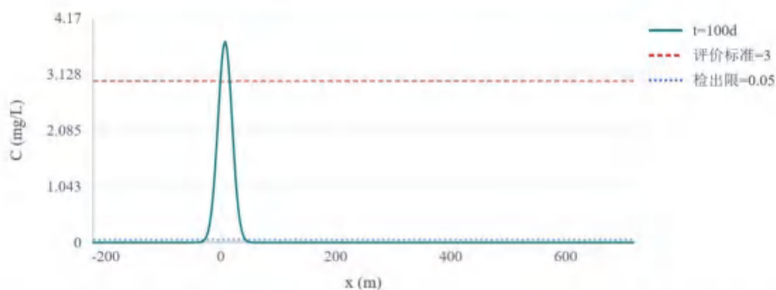
图 5.3.2-2 耗氧量 (COD Mn 法, 以 O 2 计) t=100d 地下水流向浓度变化趋势图
