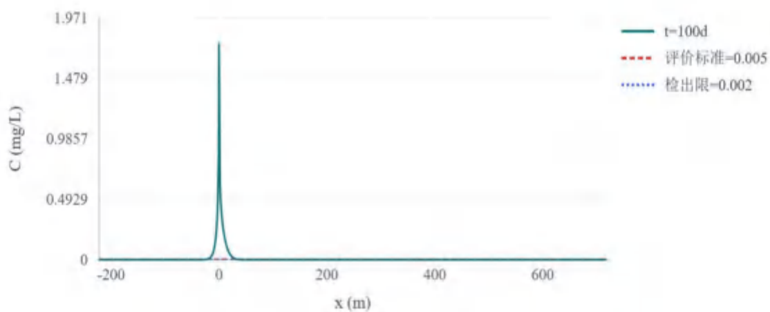
图 5.3.2-32 镉 t=100d 地下水流向浓度变化趋势图
