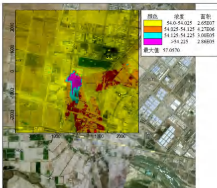
图 5.1.2-2 NO 2 保证率日均叠加浓度分布图
