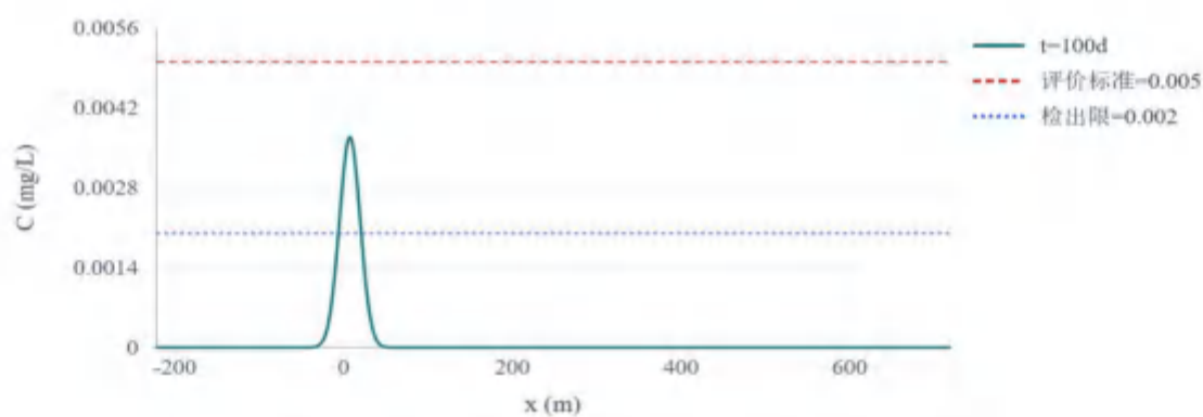
图 5.3.2-14 -镉 t=100 d 地下水流向浓度变化趋势图
