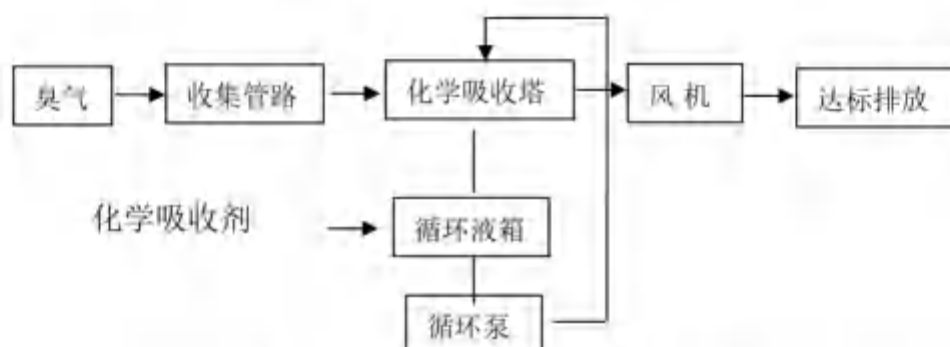
图6.1.1-5 废气处理工艺流程图
