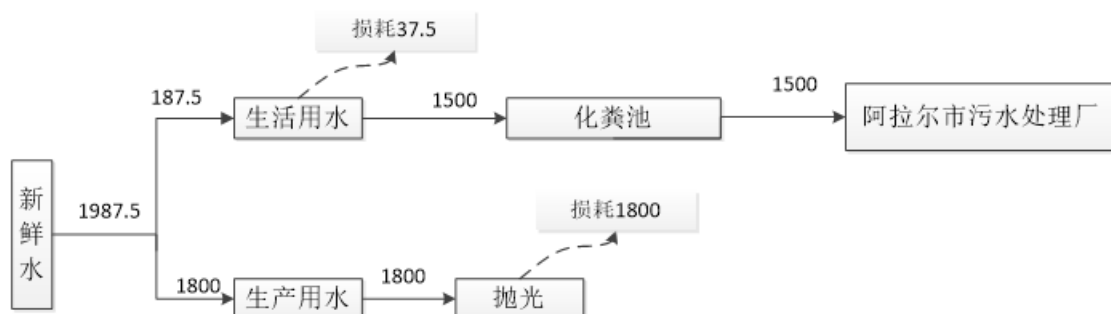
图 2-1 全厂水平衡图 单位: m³/a
