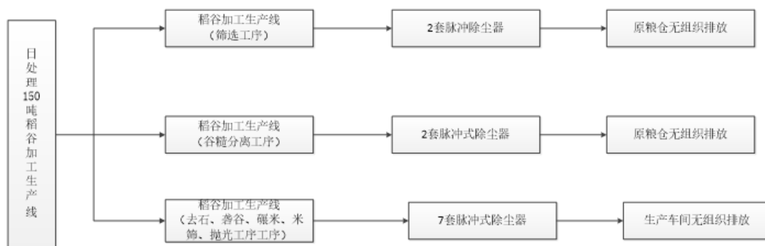
图 4-1 本项目废气处理方案
