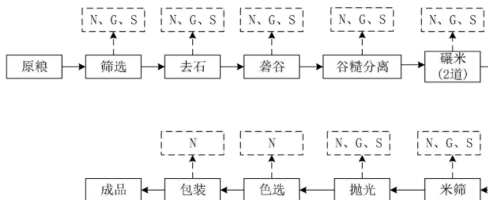
图 2-3 项目运营期生产工艺流程及产污环节示意图
