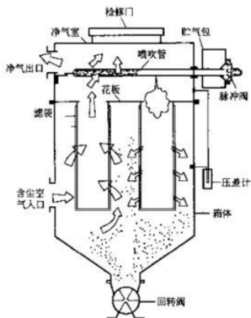
图 4-2 脉冲除尘器结构示意图
