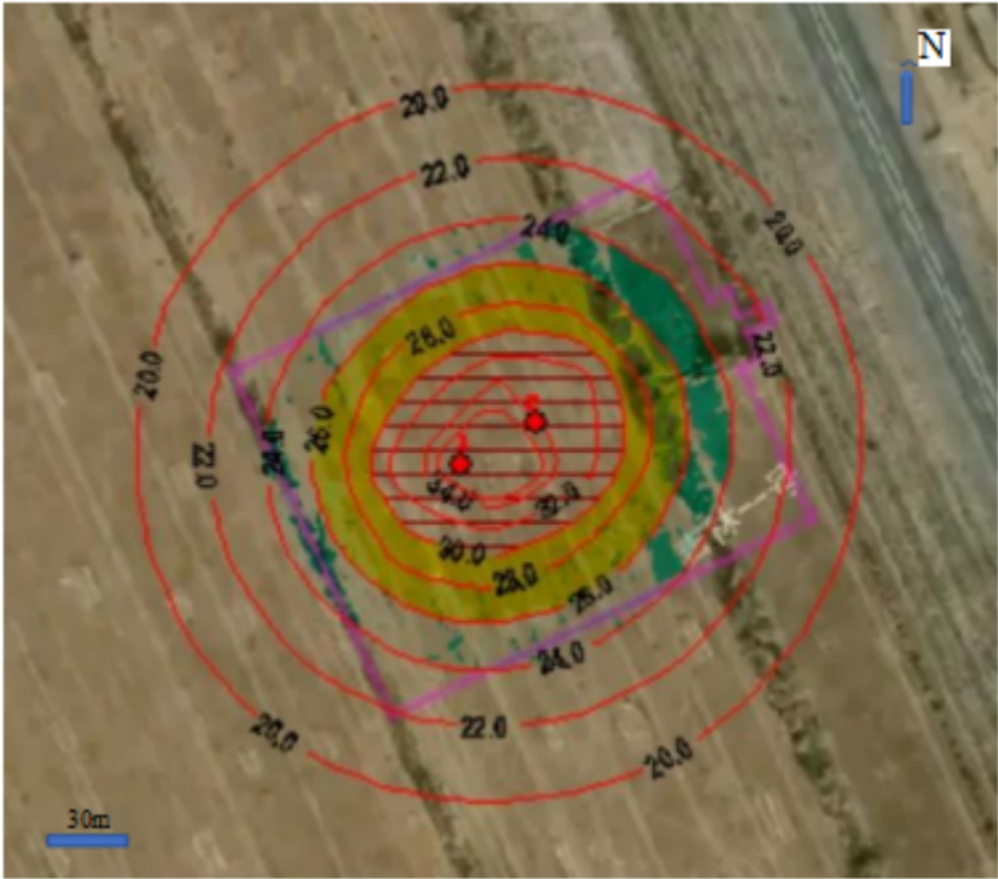
图 4-1 220kV 升压储能站等声值线图
