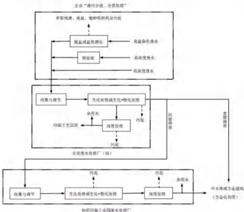
图 6.2-13 印染废水治理全流程示意图
