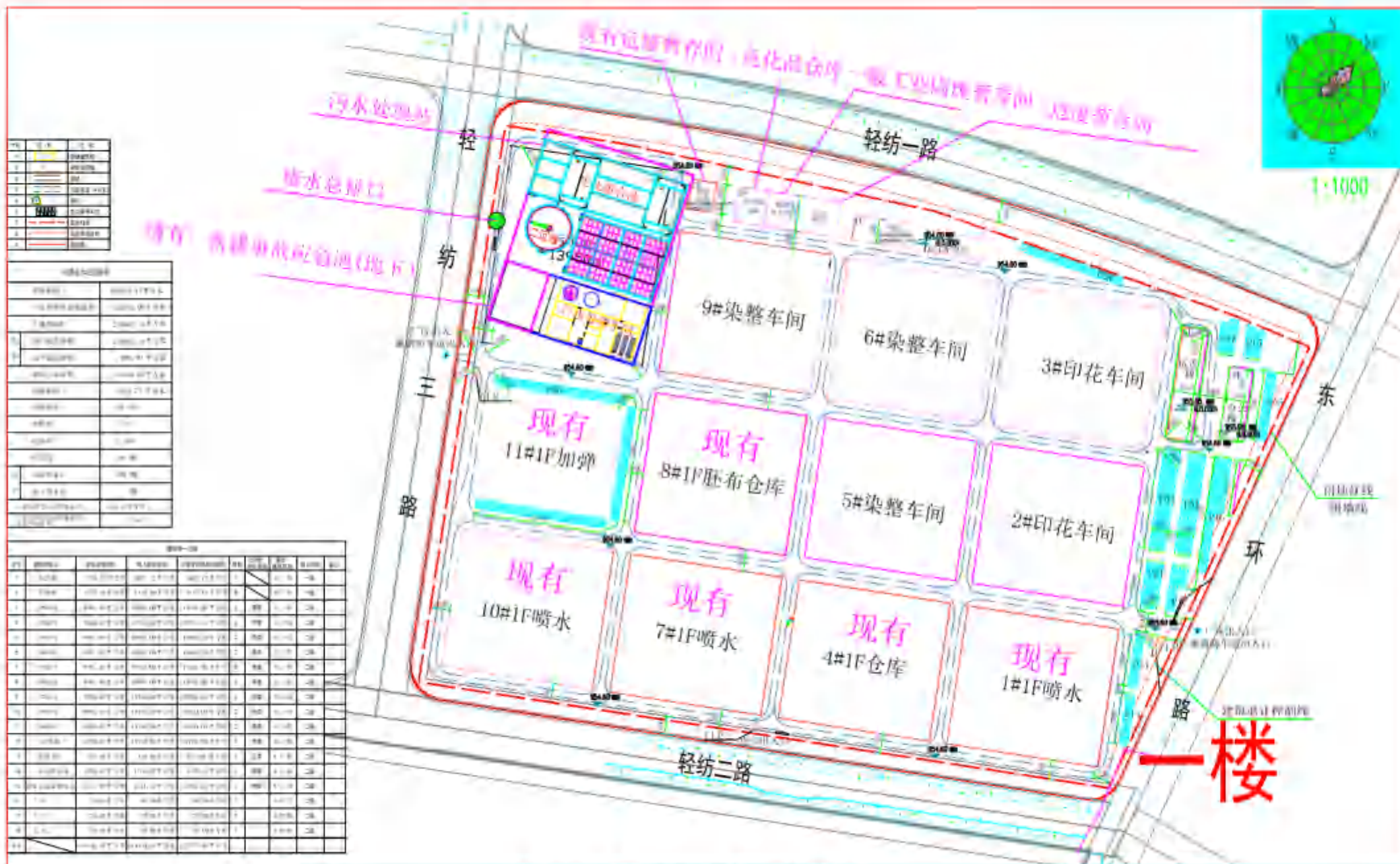
图3.1-1 本项目总平面布置示意图(一楼)
