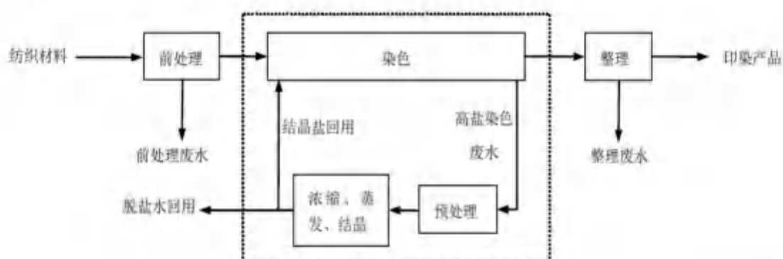
图 6.2-3 高盐染色废水结晶盐回用工艺流程示意图
