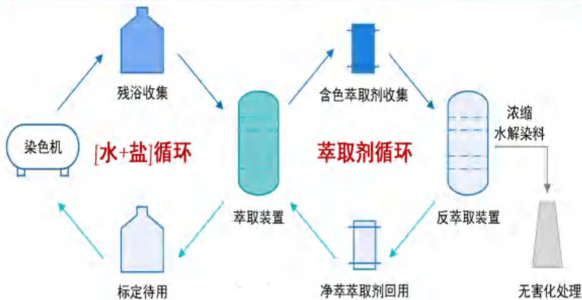
图 6.2-4 盐回用系统基本原理示意图
