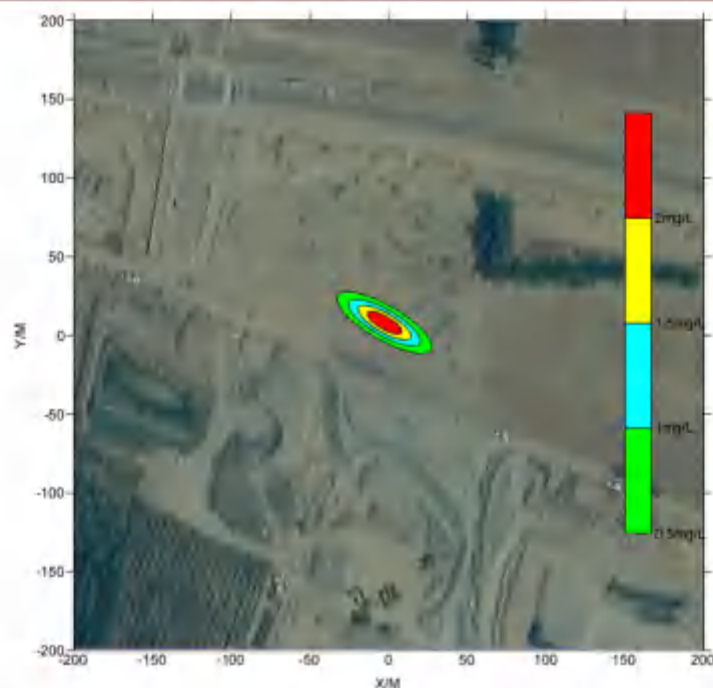
图 5.3-7 COD 短时泄露 3650d 浓度等值线图（泄漏量 10\text{m}^3 ）
