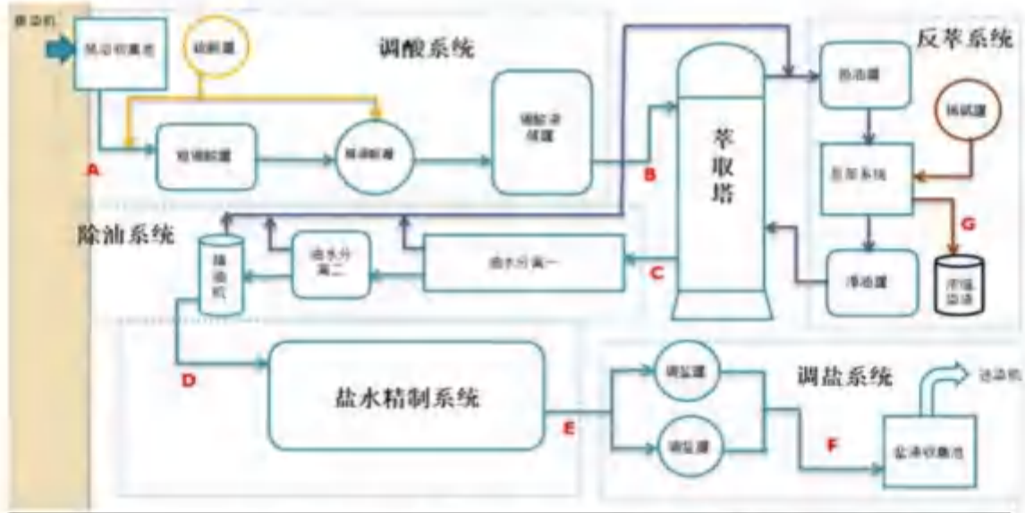
图 6.2-5 染色残液盐回用系统流程图
