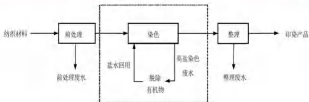
图 6.2-2 高盐染色废水盐水回用工艺流程示意图
