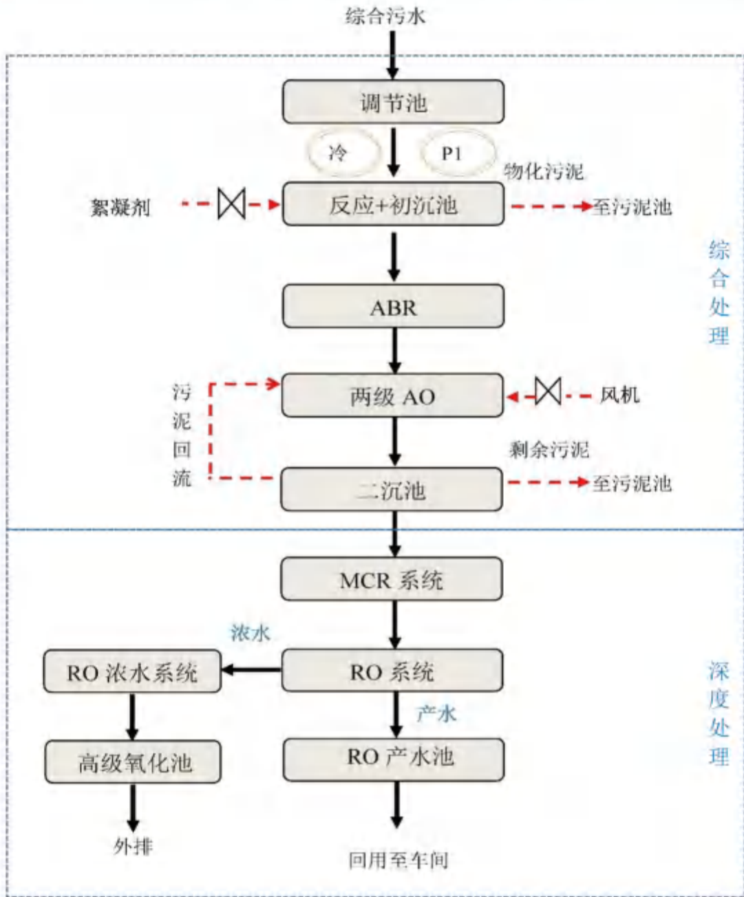
图 6.2-9 项目污水处理工艺
