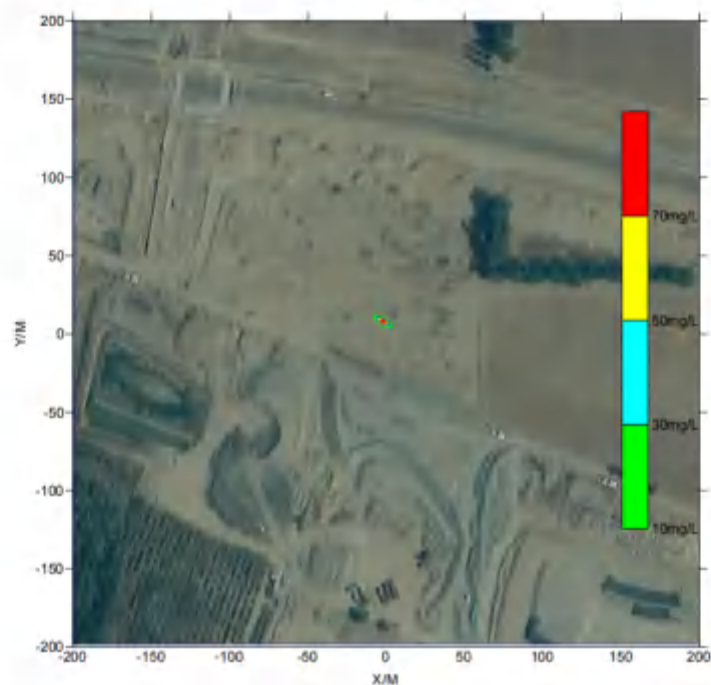
图 5.3-5 COD 短时泄露 100d 浓度等值线图（泄漏量 10\text{m}^3 ）
