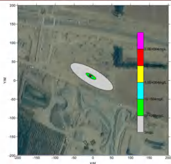
图 5.3-10 COD 长期泄露 3650d 浓度等值线图
