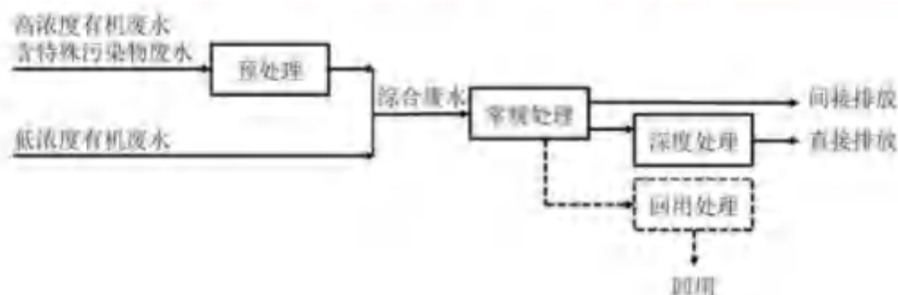
6.2-10 纺织染整工业废水治理工程技术一般工艺流程示意图
