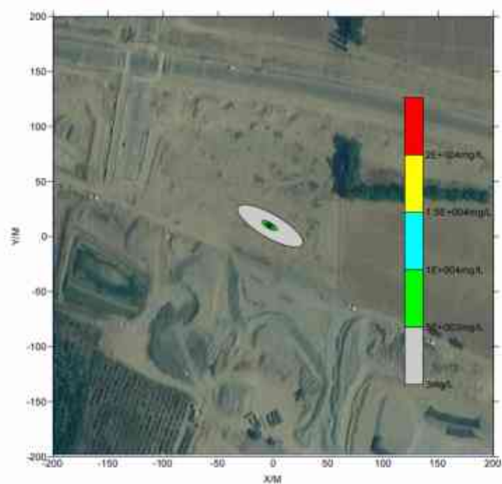
图 5.3-9 COD 长期泄露 1000d 浓度等值线图
