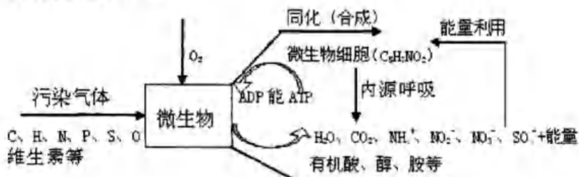
图 6.1-4 污染物的转化机理
