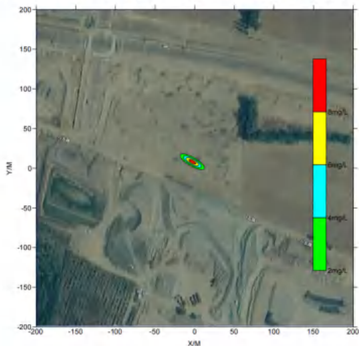
图 5.3-6 COD 短时泄露 1000d 浓度等值线图（泄漏量 10\text{m}^3 ）
