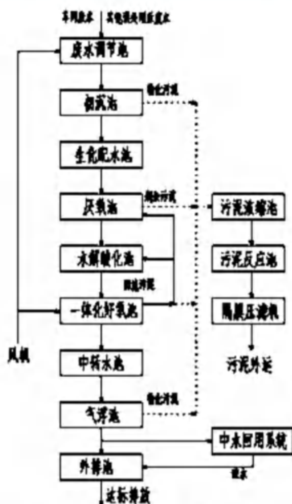
图 6.2-1 污水综合处理工艺
