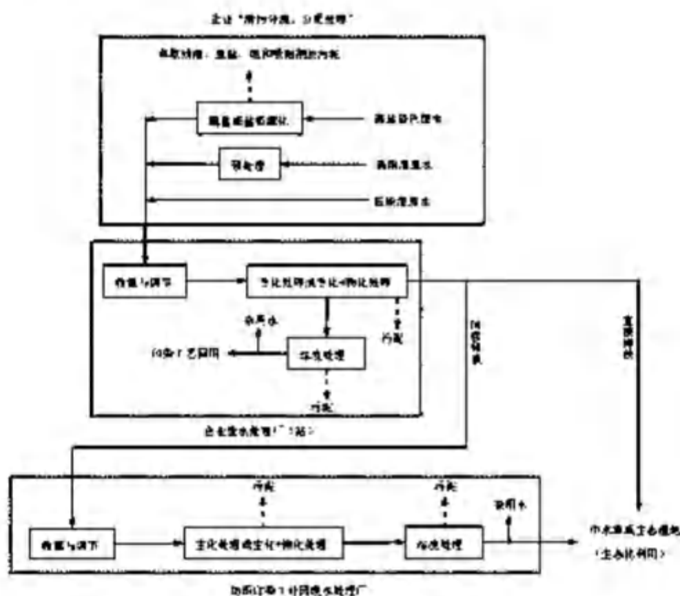
图 6.2-3 印染废水治理全流程示意图
