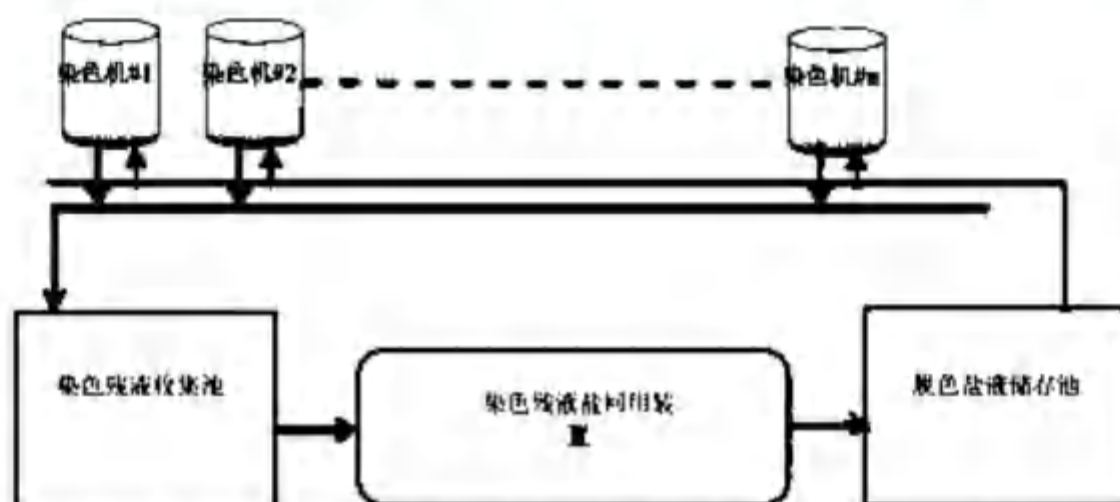
图 6.2-6 活性染料染色残液盐回用装置与染色机循环系统结构示意图
