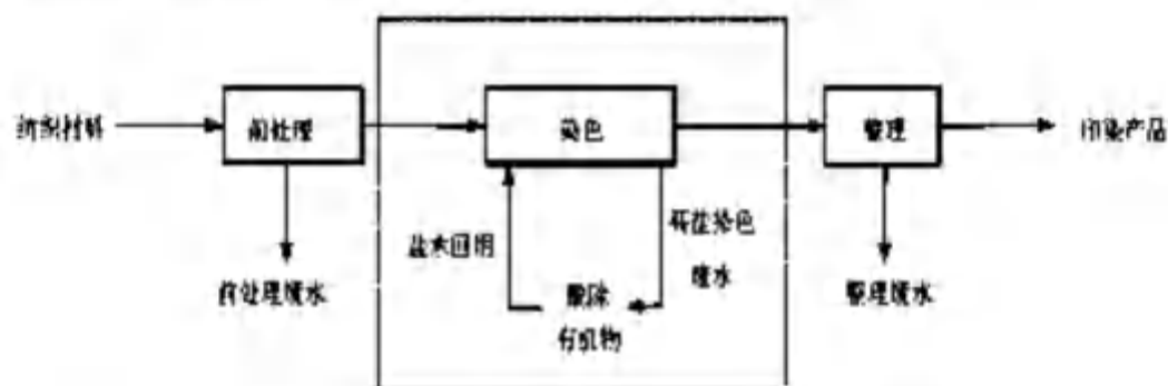
高盐染色废水盐水回用工艺流程示意图
