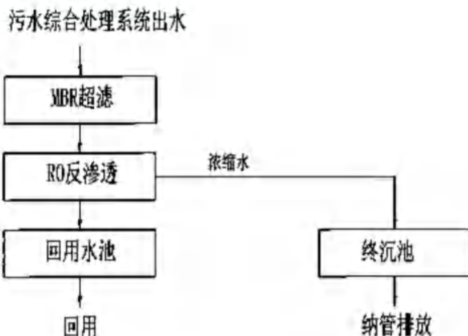
图 6.2-2 污水处理站及中水回用装置工艺流程图
