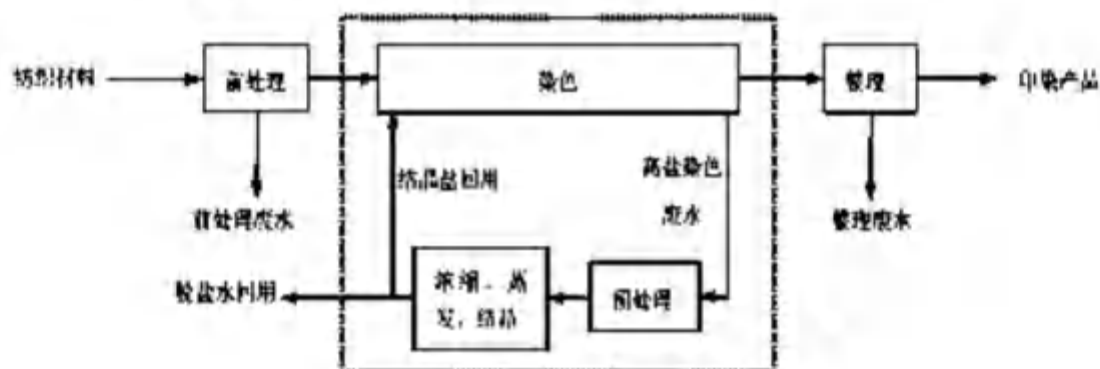
高盐染色废水结晶盐回用工艺流程示意图
