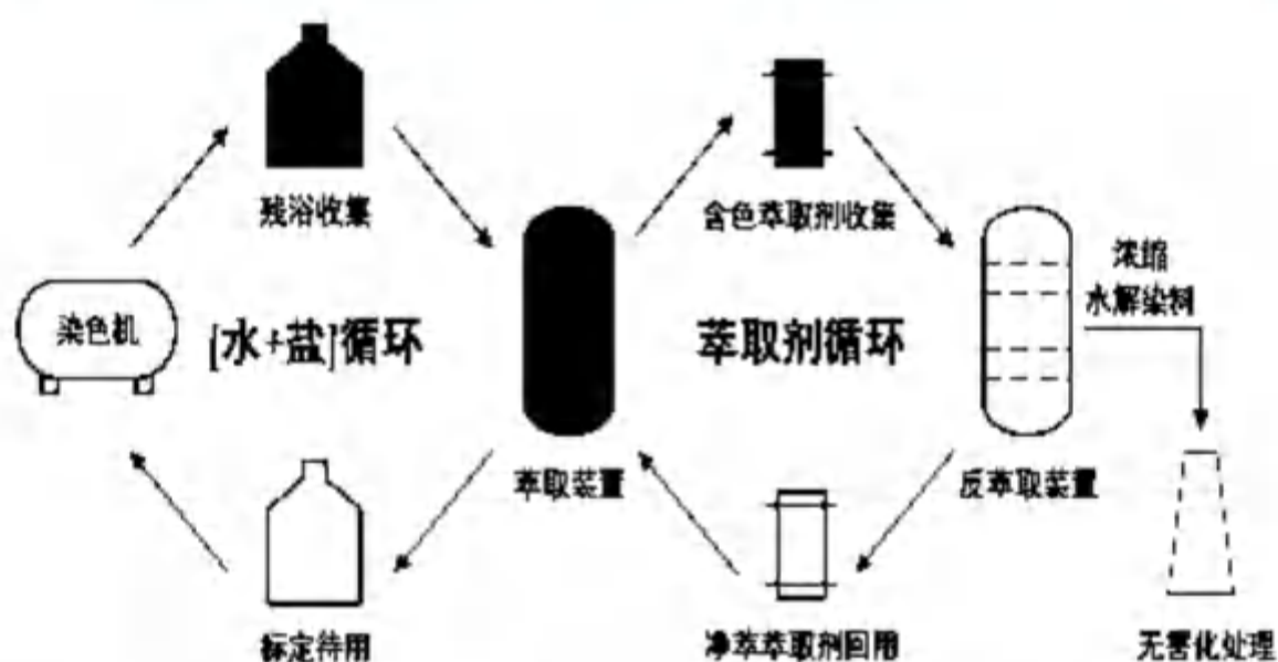
图 6.2-4 盐回用系统基本原理示意图
