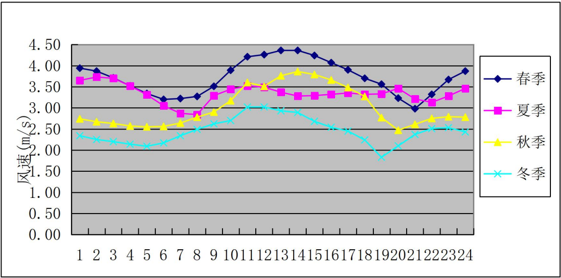
图5.1-3 阿拉尔季小时平均风速日变化曲线图
