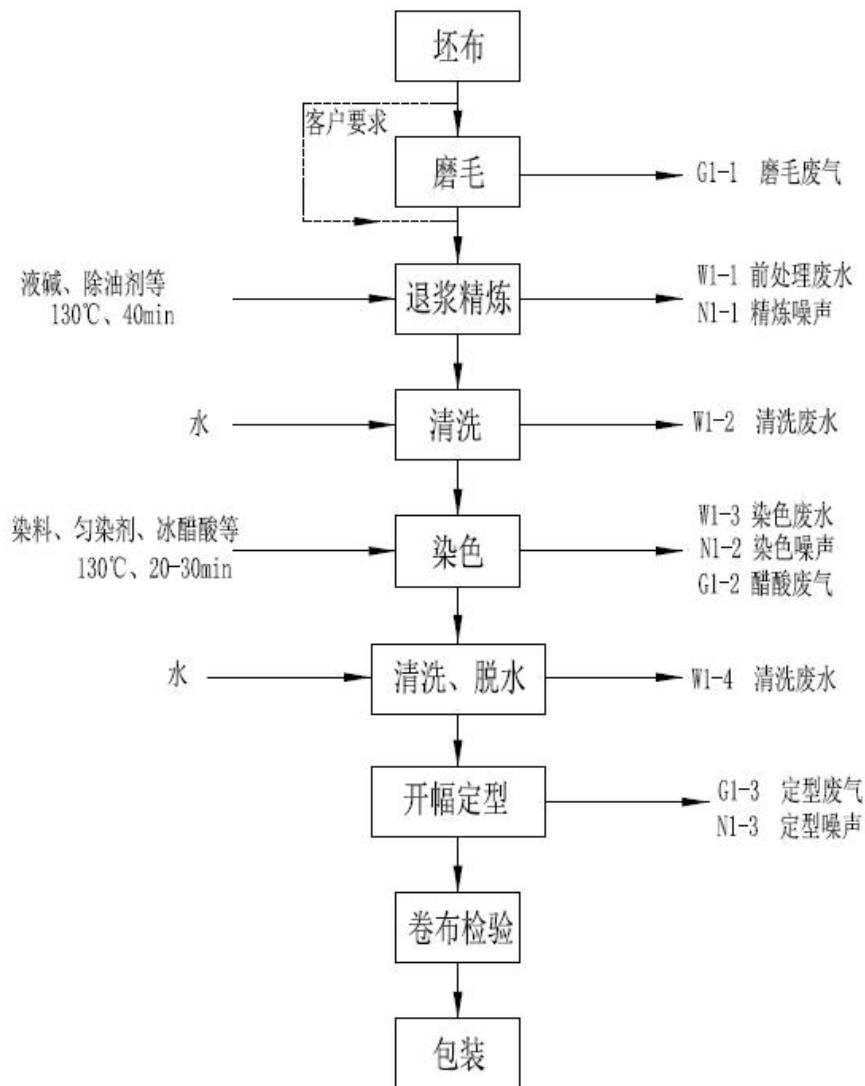
图 3.2-2 涤纶梭织布染整工艺流程及产污环节图
