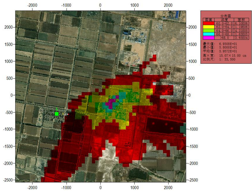
图 5.1-6 NO 2 保证率日均叠加浓度分布图
