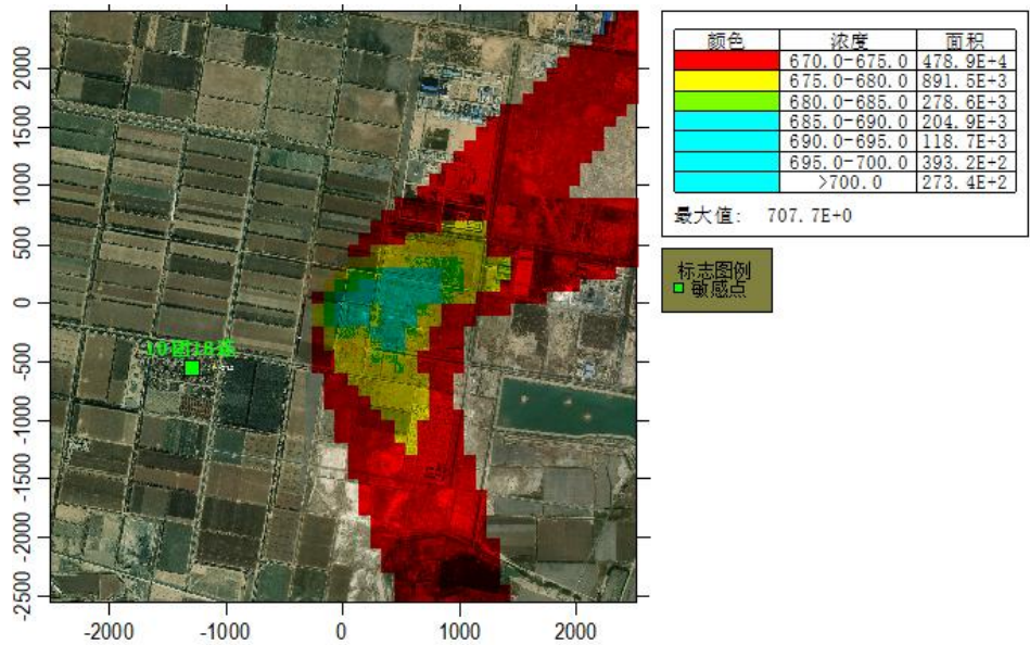
图 5.1-6 NO 2 保证率日均叠加浓度分布图
