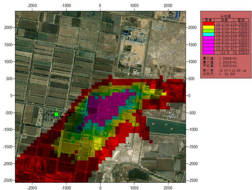
图 5.1-5 SO 2 保证率日均叠加浓度分布图
