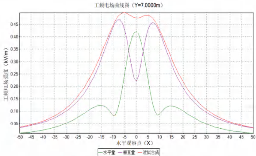
图 3.1-5 110kV 单回路线路工频电场强度预测分布曲线
