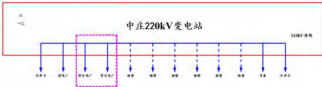
图 1 间隔平面布置图
