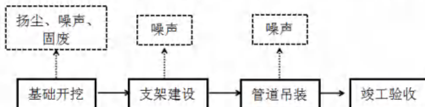
图 2 蒸汽管道工程主要施工工艺图
